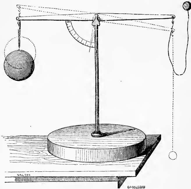
Fig. 1.— Appareil destiné à montrer qu'une force vive , directement appliquée au déplacement d'une masse, s'éteint dans un choc, tandis que la même force, transmise par un intermédiaire élastique, peut effectuer du travail. (Figure empruntée à l'ouvrage intitulé : Du Mouvement dans les fonctions de la vie , 1868).
